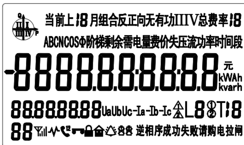
图 2 液晶全屏图
