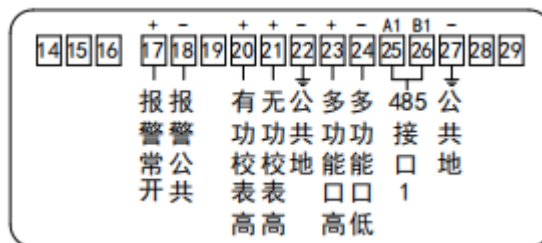
(c) 内置表
