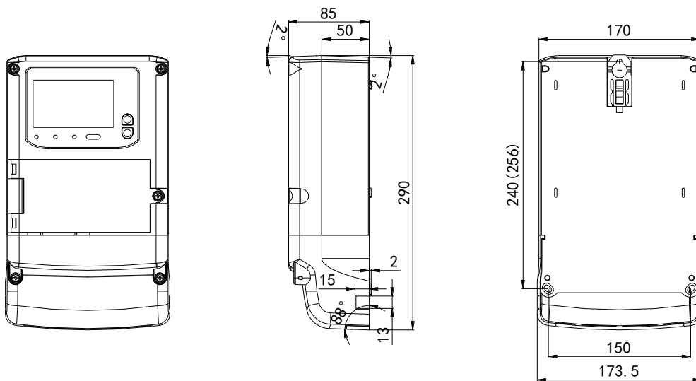
外形示意图
